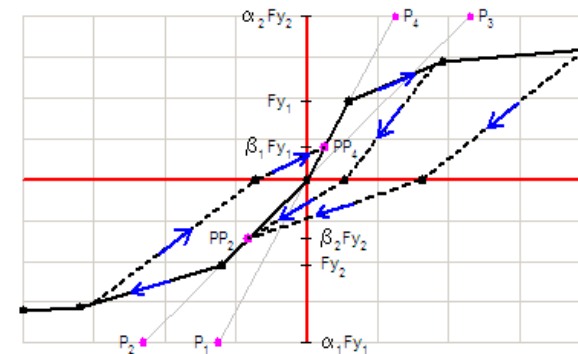
isteresi secondo il modello Pivot
