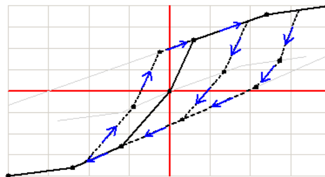
isteresi secondo un modello ad incrudimento cinematico
