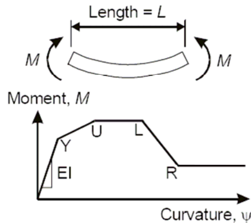
(a) Actual Beam
